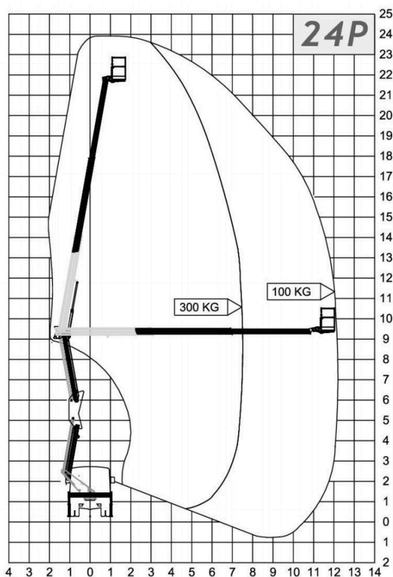
Cela Essential 24P — diagramma di lavoro
