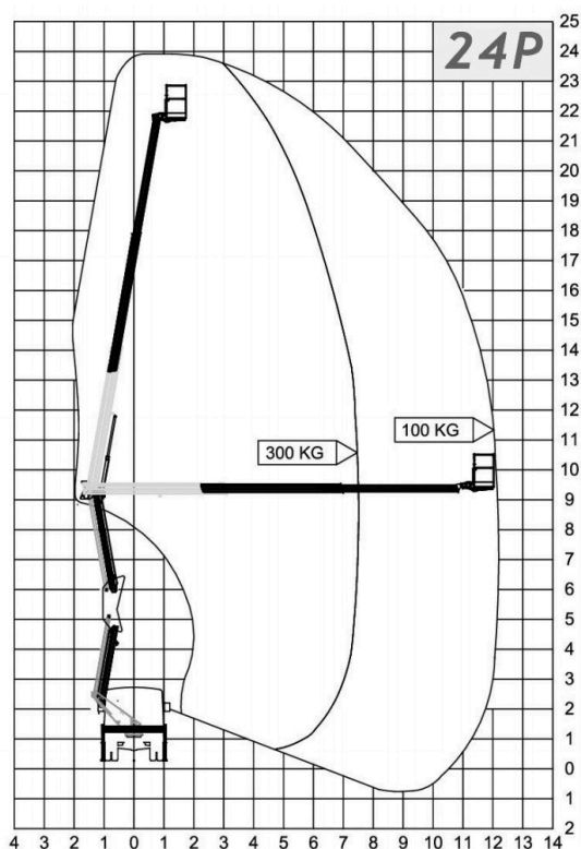
Cela Essential 24P — diagrama de trabajo
