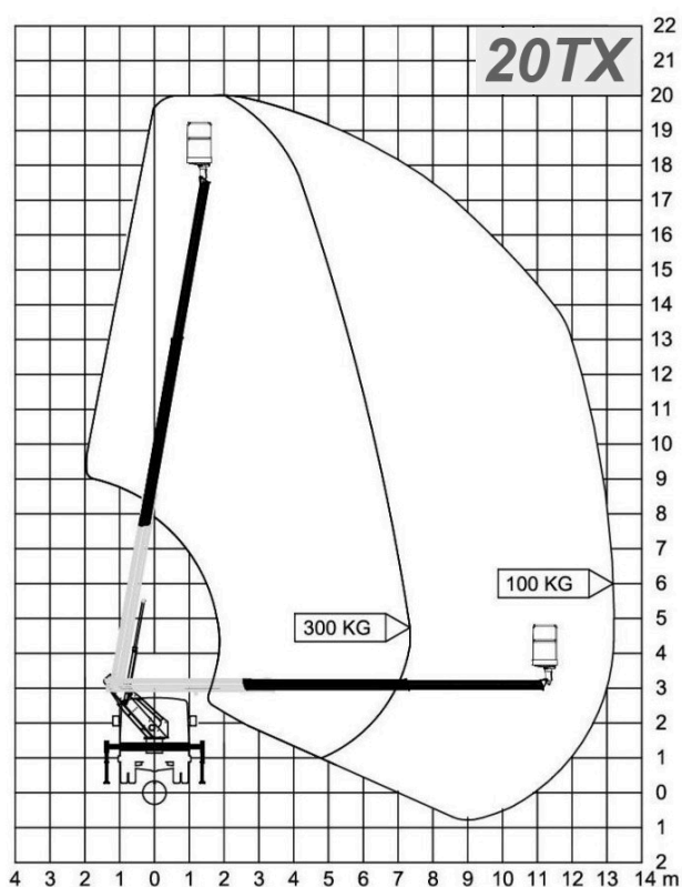
Cela Essential 20TX — diagrama de trabalho
