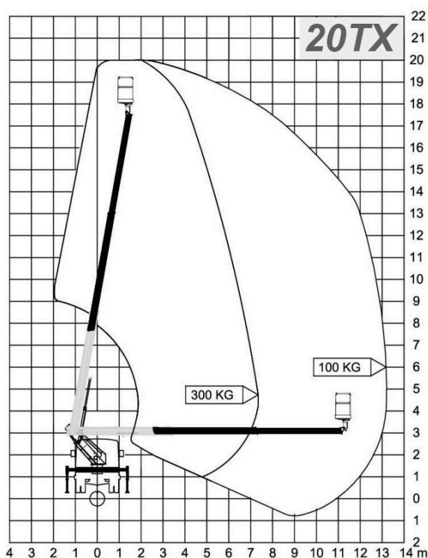
Cela Essential 20TX — diagramme de travail
