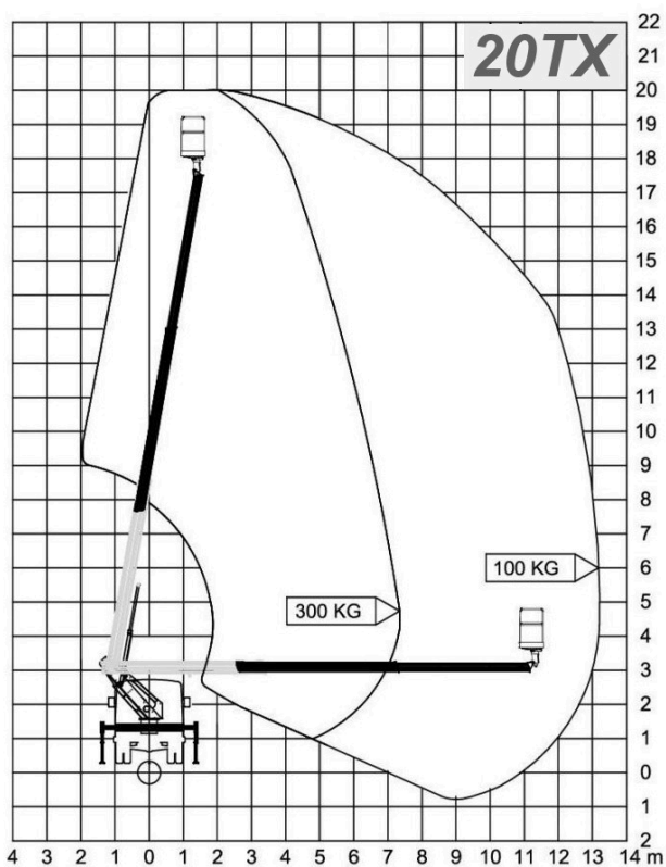
Cela Essential 20TX — διάγραμμα εργασίας
