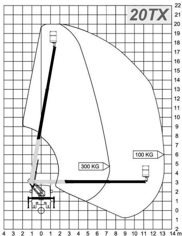
Cela Essential 20TX — pracovní diagram
