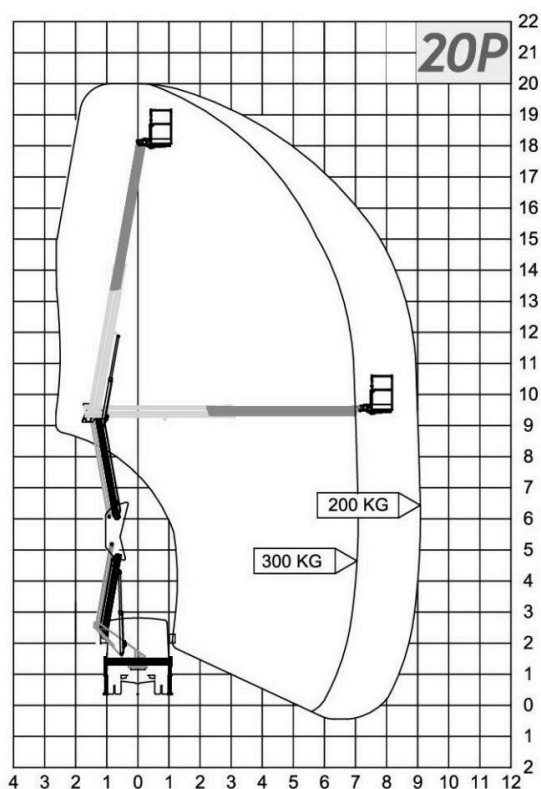
Cela Essential 20P — werkdiagram
