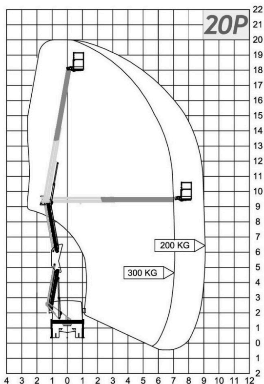
Cela Essential 20P — diagrama de trabajo
