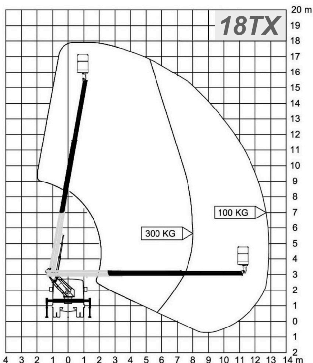
Cela Essential 18TX — διάγραμμα εργασίας
