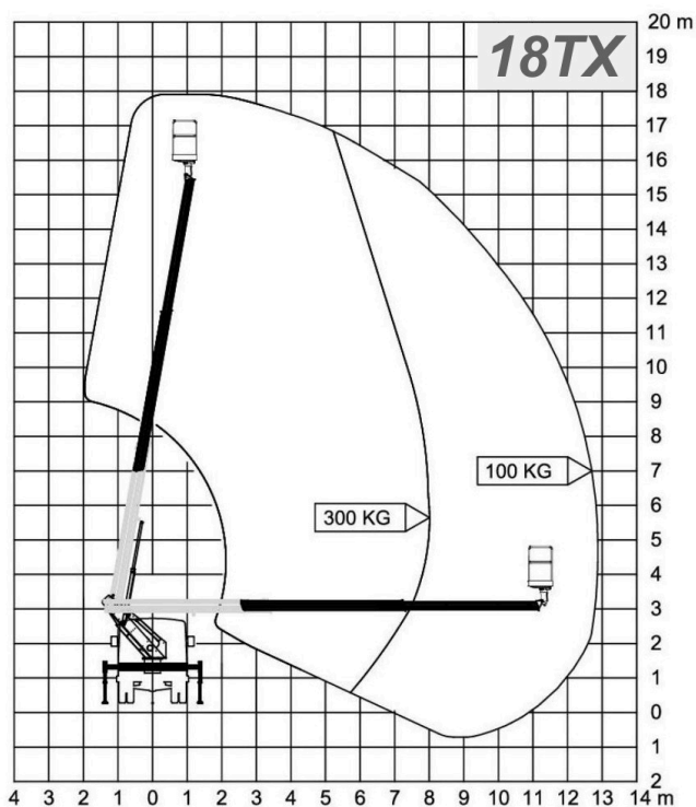
Cela Essential 18TX — Arbeitsdiagramm
