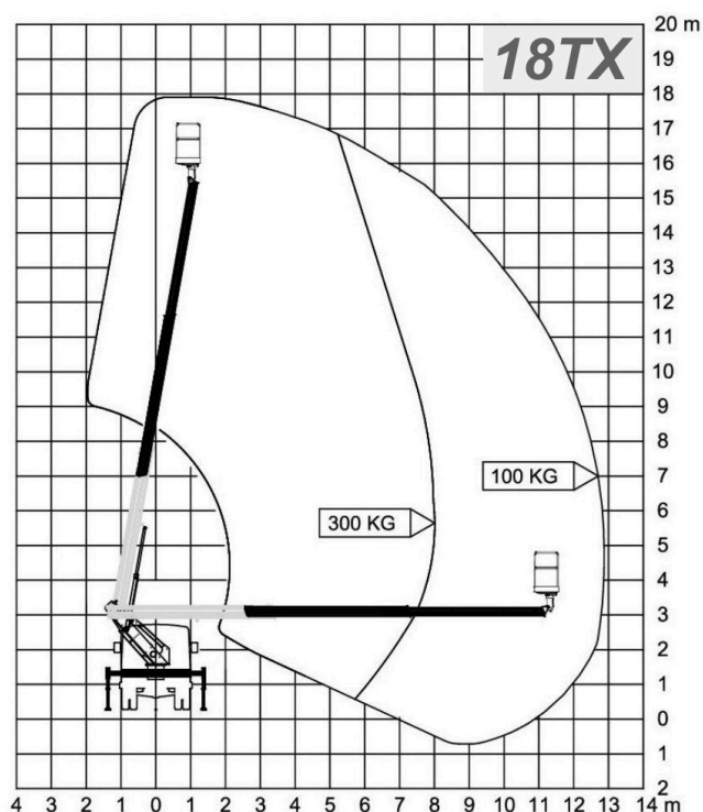
Cela Essential 18TX — arbejdsdiagram
