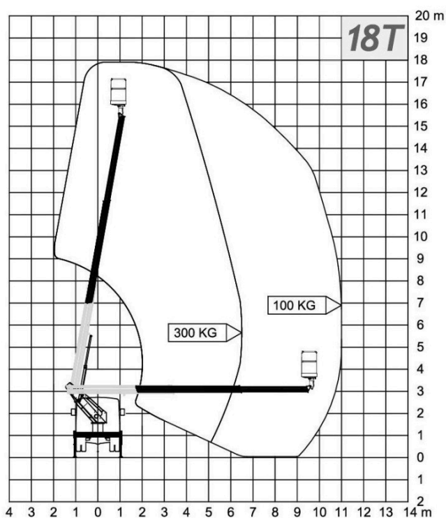
Cela Essential 18T — diagramma di lavoro
