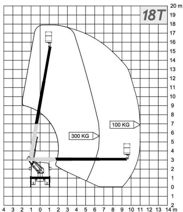
Cela Essential 18T — arbejdsdiagram
